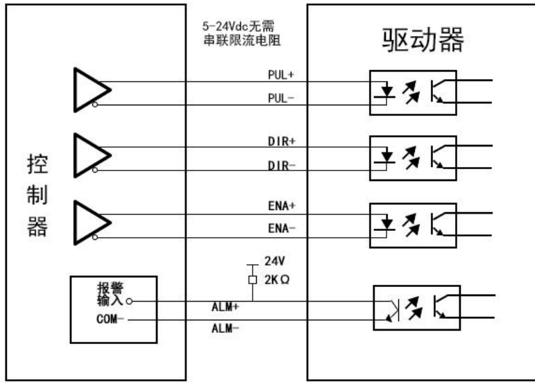
差分方式控制信号接口接线图
